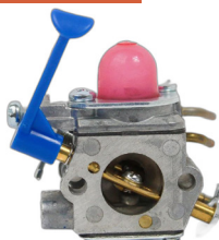
Carburador roçadeira husqv 128R/128RJ original
