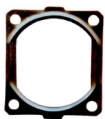
Junta cilindro stihl 066/660
