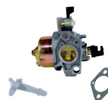
Carburador honda 11hp gx340
