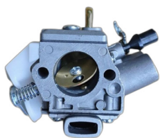
Carburador stihl 462 mod.novo
