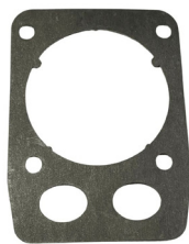
Junta cilindro roç husqv 345FR
