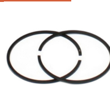
Jogo anéis pistão 34x1.5mm stihl fs 85/86/88
