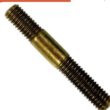
Prisioneiro filtro ar stihl 051 m5x45
